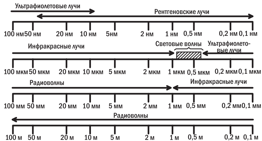
Рис. 5.12.1. Спектр частот электромагнитных колебаний
