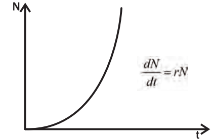
Рис. 4.4.1. Экспоненциальный рост
