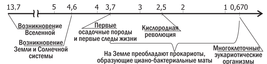
Рис. 2.10.1. Основные этапы эволюции жизни на Земле
