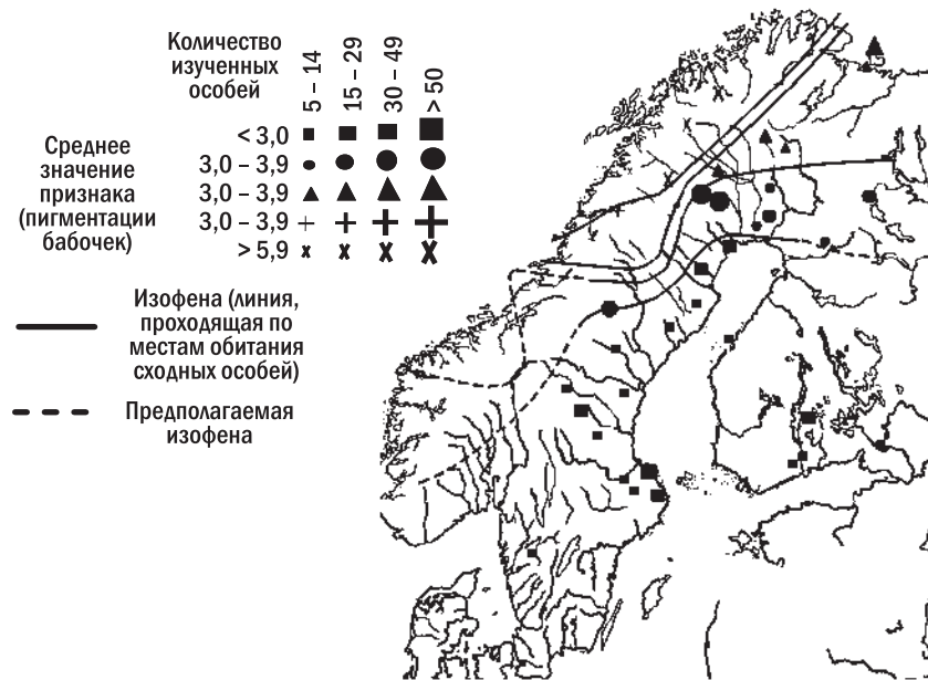
Рис. 5.21.1. На этой схеме показана клинальная изменчивость по пигментации крыльев одного из видов бабочек, брюквенниц ( Pieris napi ), по результатам исследования, выполненного в начале XX века. Изофены — линии, соединяющие области распространения организмов с одинаковой выраженностью исследуемого признака
