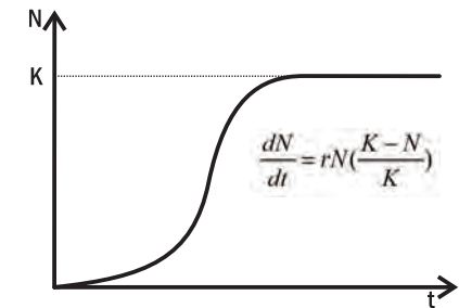
Рис. 4.4.2. Логистический рост
